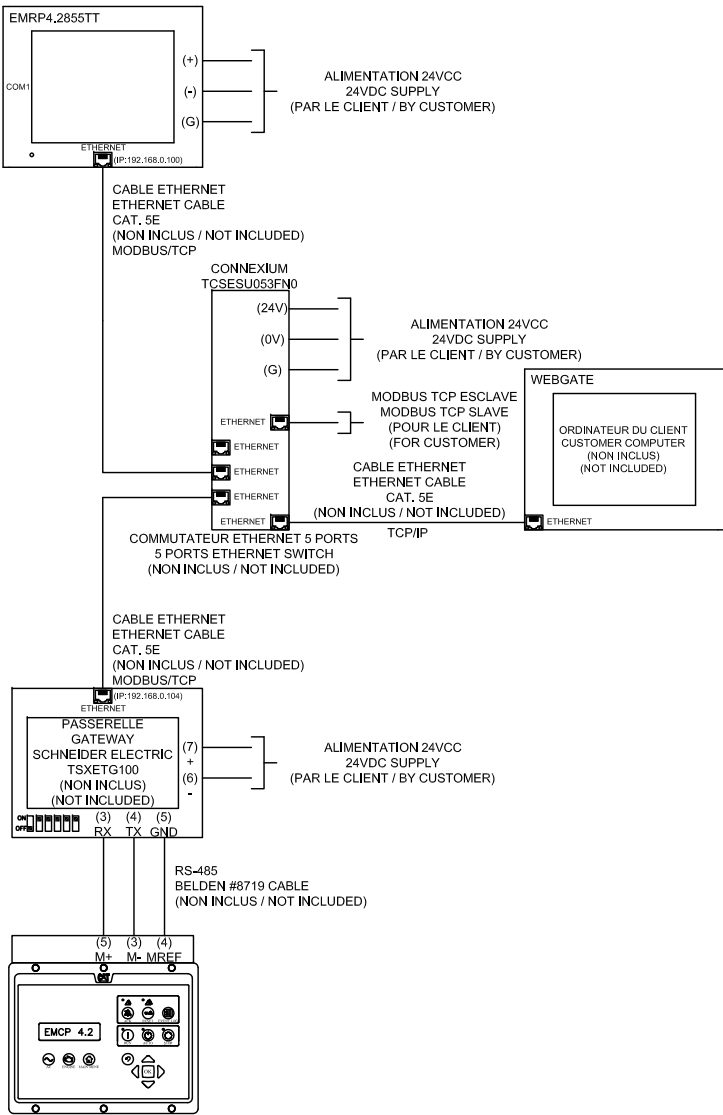
EMRP4.2855TT CONFIGURATION OPTIONNELLE OPTIONAL SETUP
