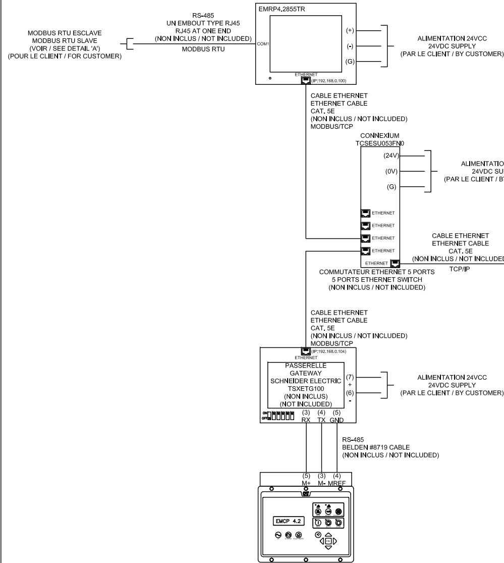
EMRP4.2855TR CONFIGURATION OPTIONNELLE OPTIONAL SETUP
